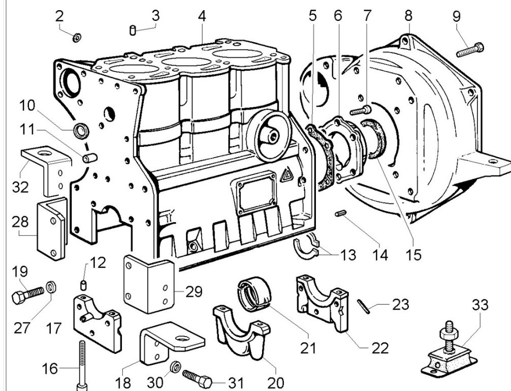
MOTORE: LDW 1003 M - TAVOLA: E
