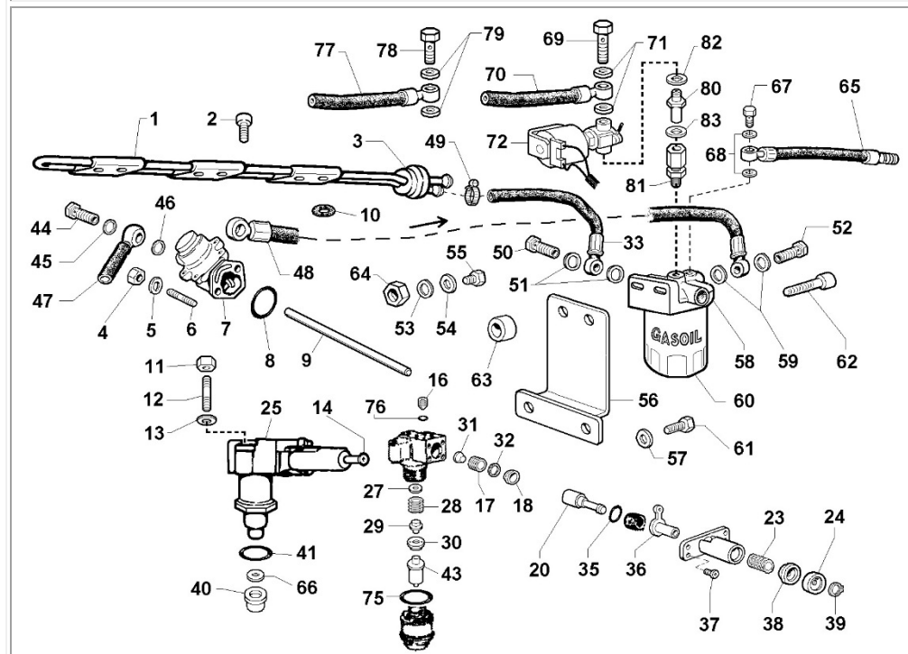
MOTORE: LDW 1003 M - TAVOLA: F
